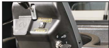
Der Ladestecker wird an die 3-polige Ladebuchse an der Lenksäule angeschlossen. Die Ladebuchse befindet sich unter der Schutzklappe.
